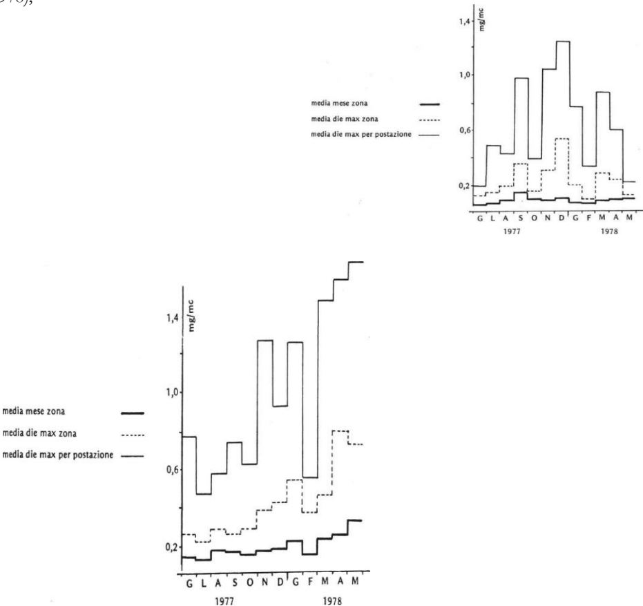
Fig. 11 ( pag. prima in basso ) Rete di rilevamento Montedison di SO2 nella zona industriale (1977–1978);
